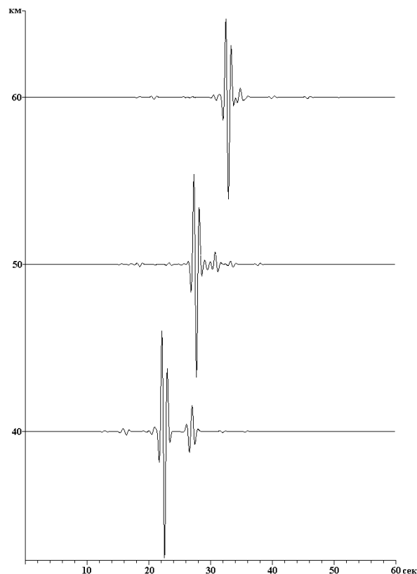
Рис. 2. Расчет минутной записи компоненты u_z для модели Луны без зоны малых скоростей (реголита). Приемники расположены на расстоянии 40, 50 и 60 км от источника.
